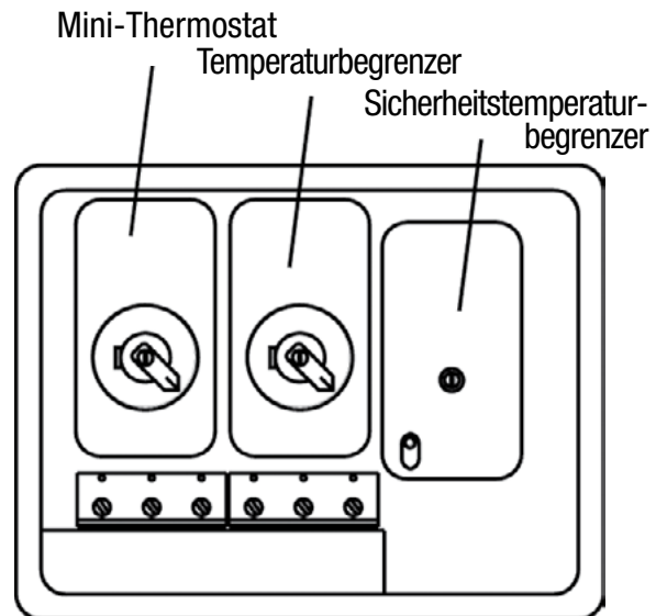
Dreifachthermostat Innenansicht
