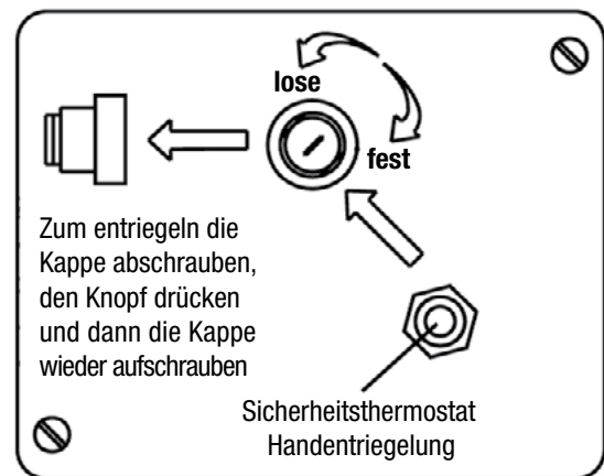
Dreifachthermostat Aussenansicht
